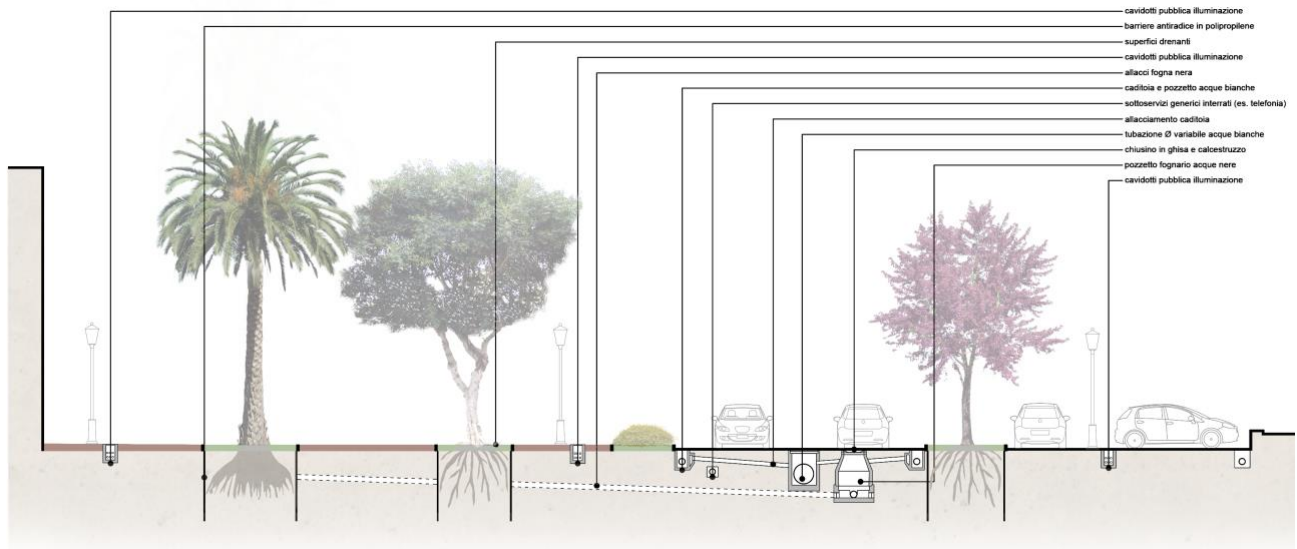
Sezione tipo sul corso Cavour – opere manutentive impiantistiche
